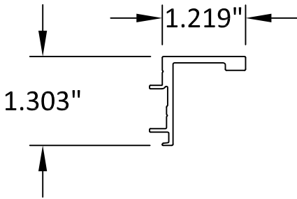
2 FRAME JAMB 6063-T5
